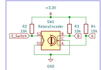
Encoder breakout module
